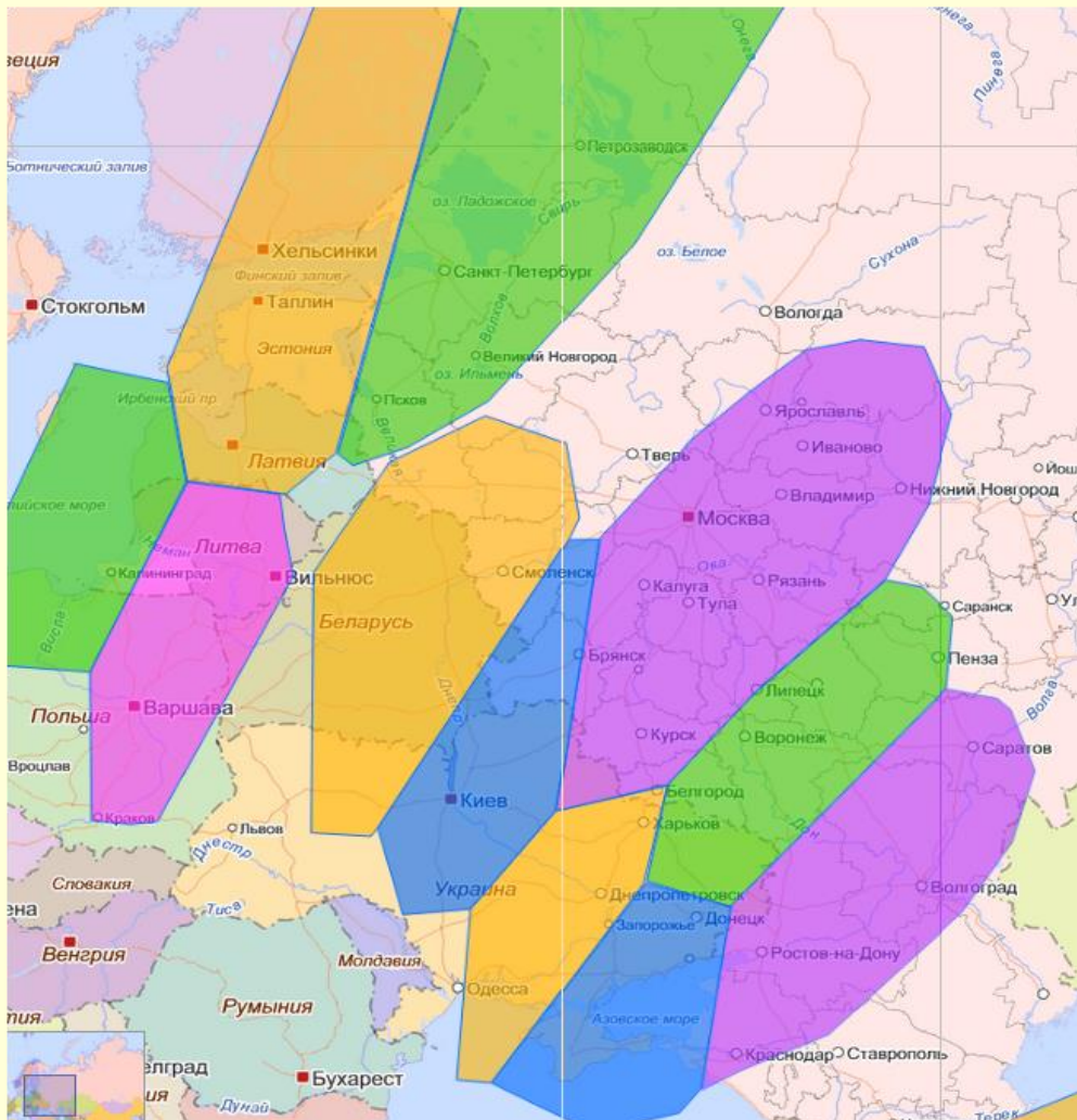
Зона покрытия спутника Ka-Sat (9E)
